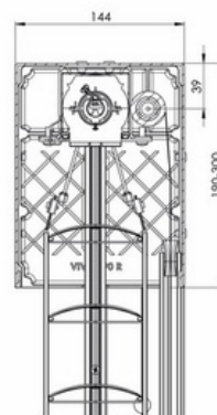
Dwarsdoorsnede van de zichtbare zelfdragende jaloezie
